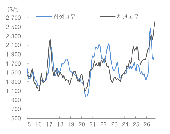
그림 111. 고무가격
