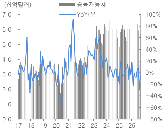
그림 36. 승용차 수출액
