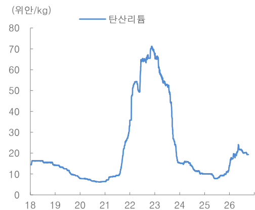
그림 105. 리튬 가격
