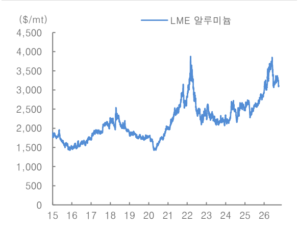
그림 102. 알루미늄 가격
