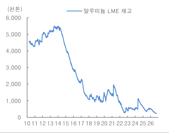
그림 109. 알루미늄 재고
