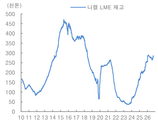
그림 108. 니켈 재고
