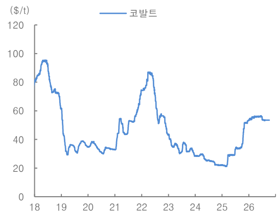
그림 106. 코발트 가격
