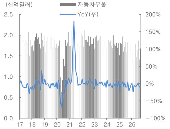
그림 37. 부품 수출액
