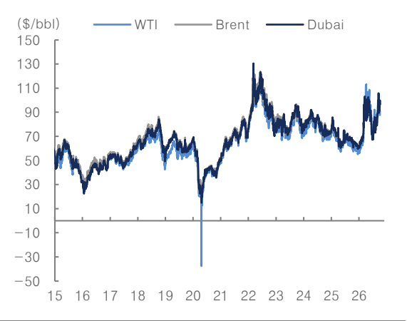
그림 110. 원유 가격
