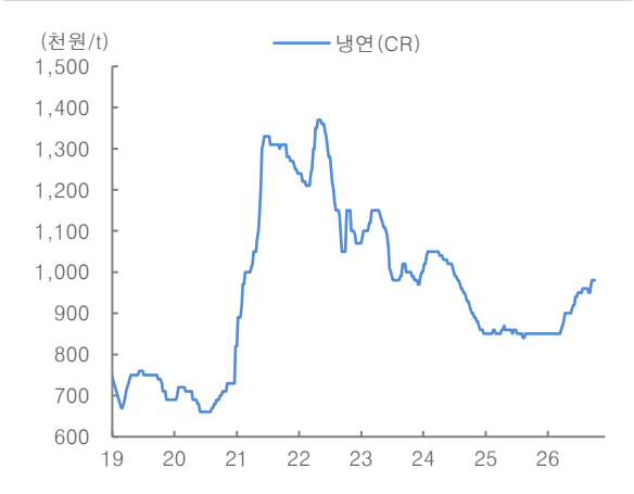
그림 101. 강판 가격
