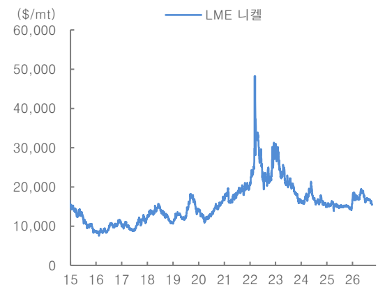
그림 104. 니켈 가격
