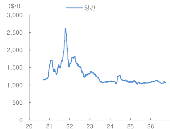
그림 107. 망간 가격
